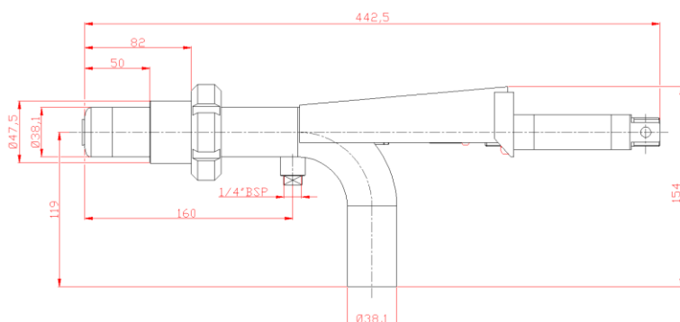
VÁLVULA COLETORA DE AMOSTRA MANUAL CÓDIGO: 4390-00
