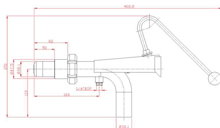
VÁLVULA COLETORA DE AMOSTRA MANUAL CÓDIGO: 4390-00
